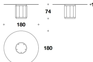
RTB (25) TAVOLO / TABLE Ø 180x74H. - THK.1cm Ø 71x29H. - THK.6/16"
