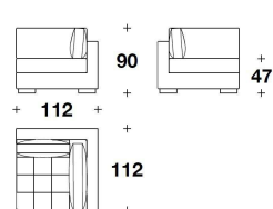
SHT (ANG) ELEMENTO ANGOLARE / CORNER ELEMENT 112x112x90H. - H.S.47 cm 44x44x35 1/3H. - H.S.18 2/4 "
