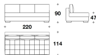
SHT (E3C) ELEMENTO 3 POSTI CENTRALE / 3 SEATER CENTRAL ELEMENT 220x114x90H. - H.S.47 cm 86 2/3x45x35 1/3H. - H.S.18 2/4 "
