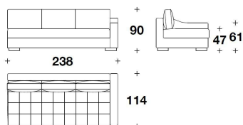
SHT (E3DB) - SHT (E3SB) ELEMENTO 3 POSTI CON BRACCIOLO DX O SX / 3 SEATER ELEMENT WITH RIGHT OR LEFT ARMREST 238x114x90H. - H.A.61 - H.S.47 cm 93 2/3x45x35 1/3H. - H.A.24 - H.S.18 2/4 "
