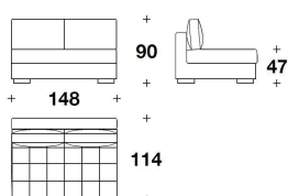
SHT (E2C) ELEMENTO 2 POSTI CENTRALE / 2 SEATER CENTRAL ELEMENT 148x114x90H. - H.S.47 cm 58 1/3x45x35 1/3H. - H.S.18 2/4 "
