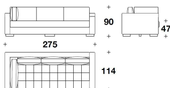
SHT (E3ADB) - SHT (E3ASB) ELEMENTO ANGOLARE 3 POSTI SX/DX CON BRACCIOLO DX/SX / LEFT OR RIGHT 3 SEATER CORNER ELEMENT W/RIGHT OR LEFT ARMREST 275x114x90H. - H.A.61 - H.S.47 cm 108 1/3x45x35 1/3H. - H.A.24 - H.S.18 2/4 "
