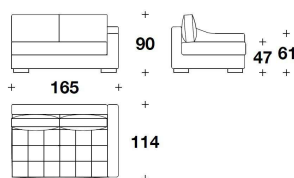
SHT (E2DB) - SHT (E2SB) ELEMENTO 2 POSTI CON BRACCIOLO DX O SX / 2 SEATER ELEMENT WITH RIGHT OR LEFT ARMREST 165x114x90H. - H.A.61 - H.S.47 cm 65x45x35 1/3H. - H.A.24 - H.S.18 2/4 "
