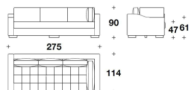
SHT (E3ADB) - SHT (E3ASB) ELEMENTO ANGOLARE 3 POSTI SX/DX CON BRACCIOLO DX/SX / LEFT OR RIGHT 3 SEATER CORNER ELEMENT W/RIGHT OR LEFT ARMREST 275x114x90H. - H.A.61 - H.S.47 cm 108 1/3x45x35 1/3H. - H.A.24 - H.S.18 2/4 "
